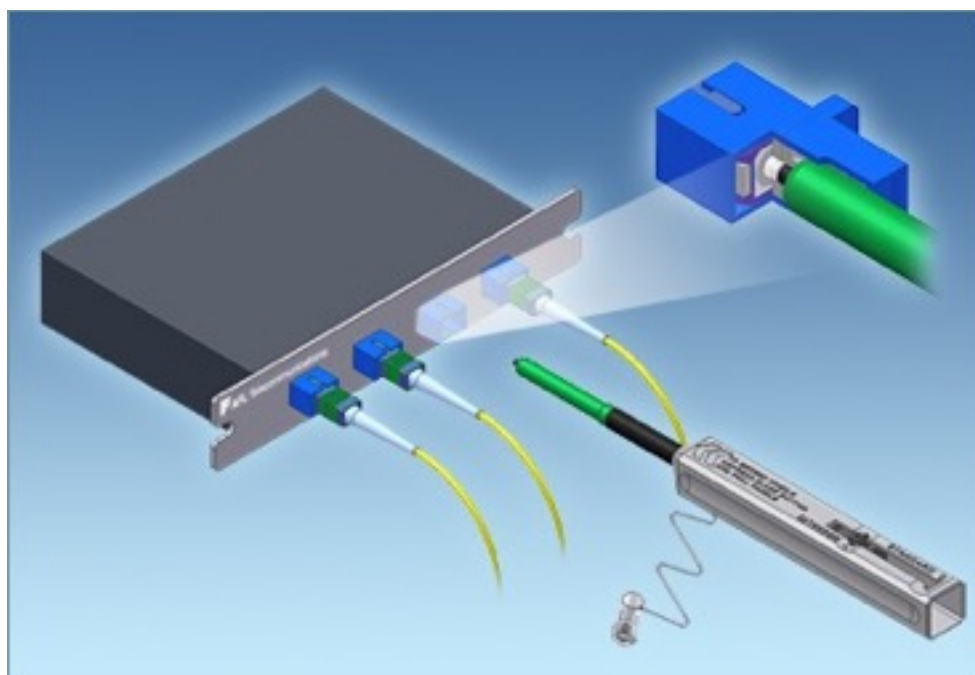
メス側コネクタ清掃図
